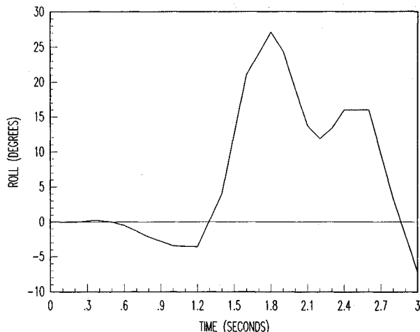
b) Roll vs time
